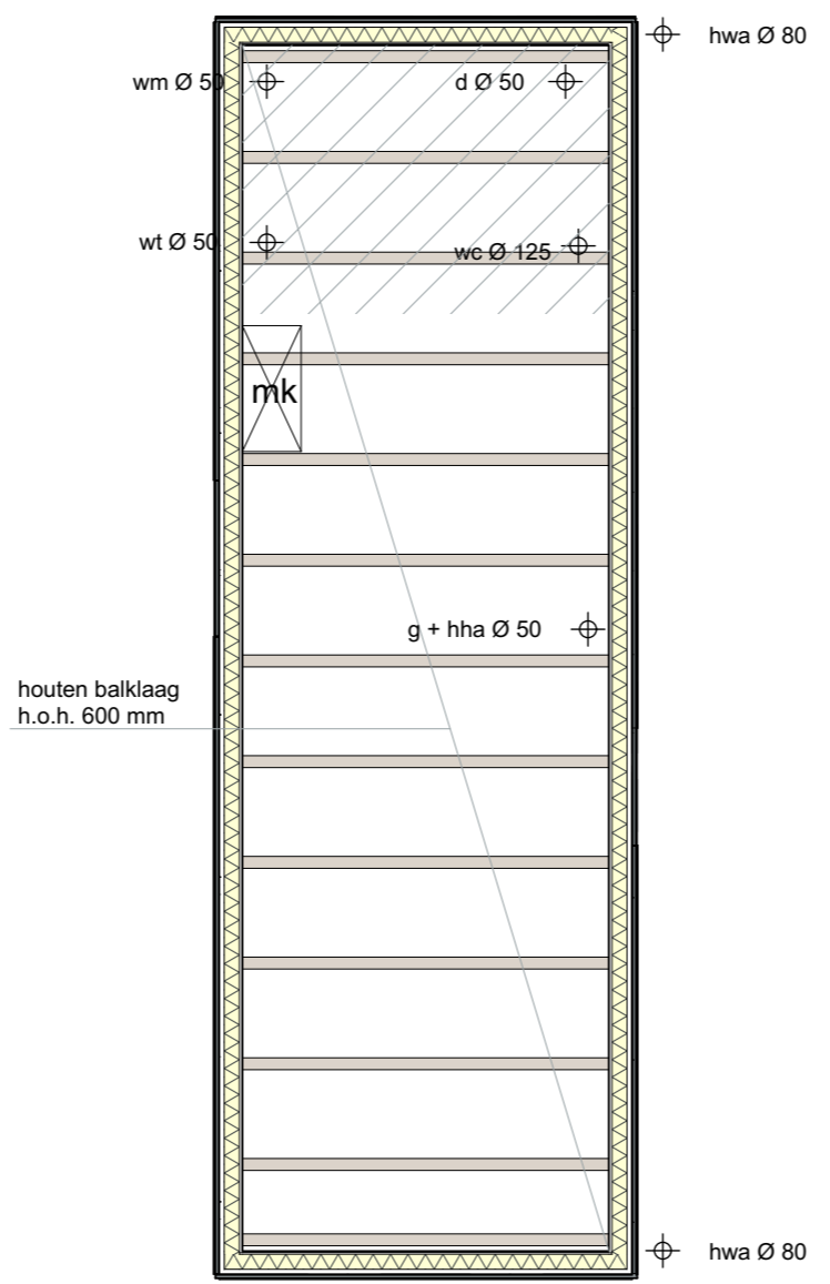
begane grondvloer
